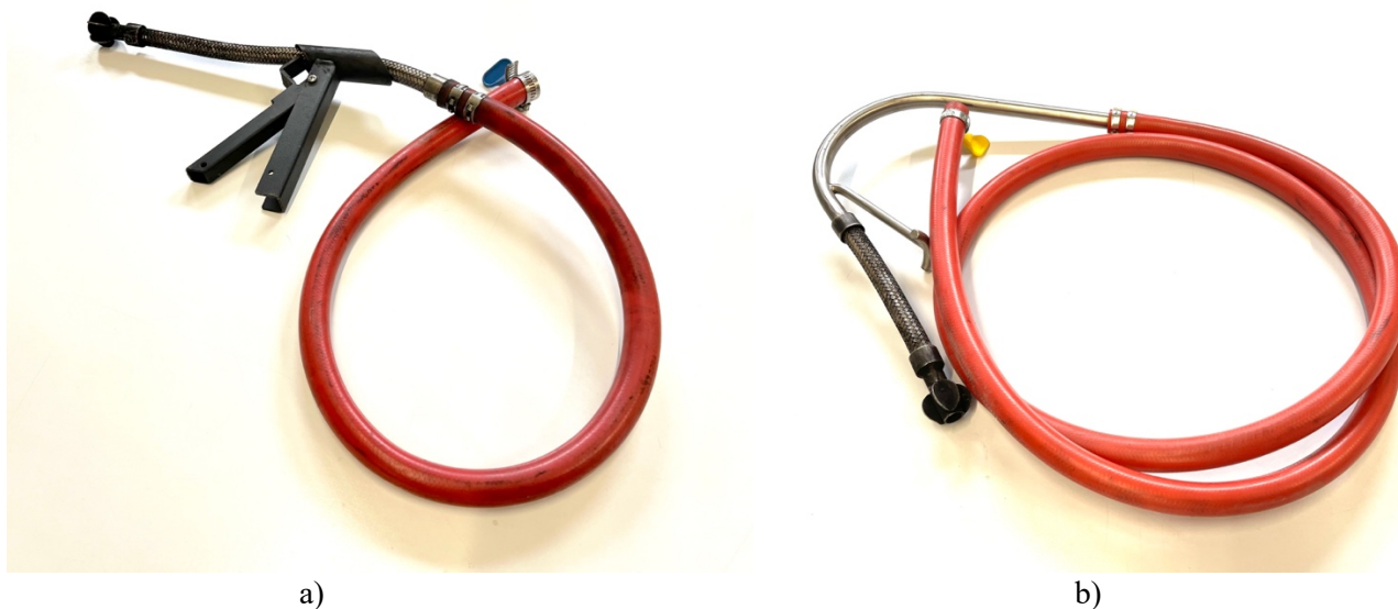
Obr. 1 Odberové sondy dymomeru ACTIA/ATAL AT 605 a) s priemerom 10 mm a dĺžkou prírodného potrubia 1149 mm b) s priemerom 10 mm a dĺžkou prírodného potrubia 1900 mm (traktorová)
